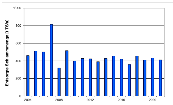
Abb. 18: entsorgte Schlammengen
