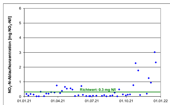
Abb. 15: Nitrit-Konzentration
