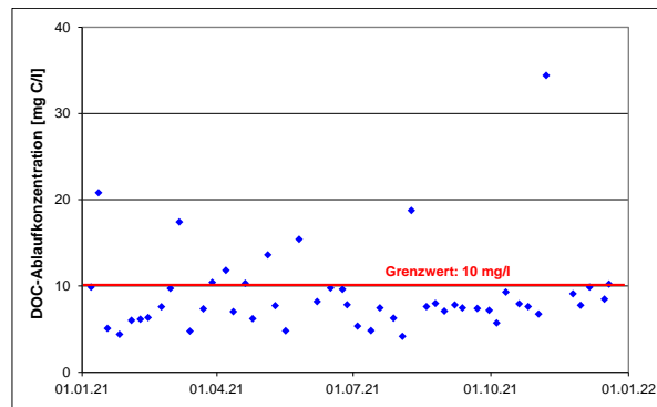
Abb. 11: DOC-Konzentration
