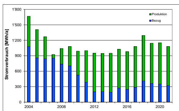
Abb. 19: Stromeigenproduktion und -einkauf
