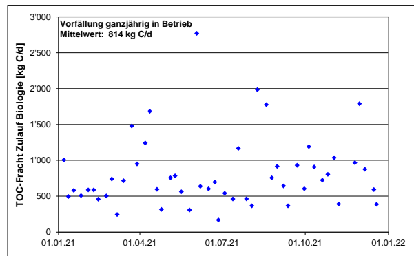
Abb. 7: TOC-Fracht Zulauf Biologie
