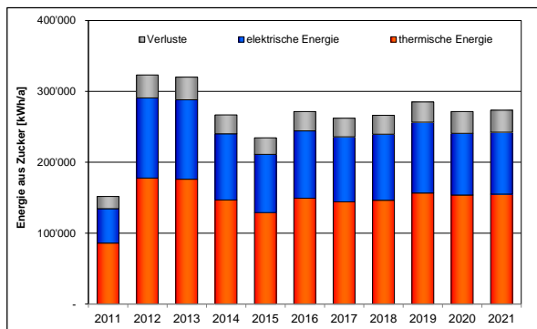
Abb. 21: Energieproduktion aus Ausschuss-Zucker
