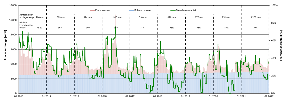
Abb. 16: Fremdwasseranfall Zulauf ARA-Zwingen
