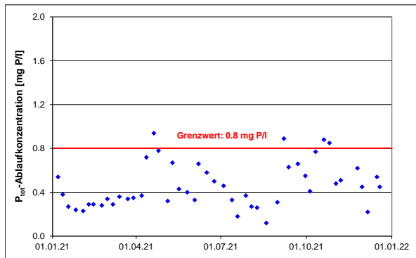
Abb. 12: Phosphor-Konzentration
