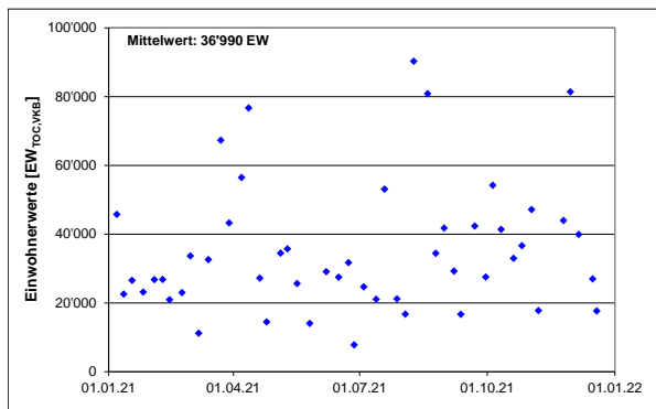
Abb. 8: Belastung ARA
