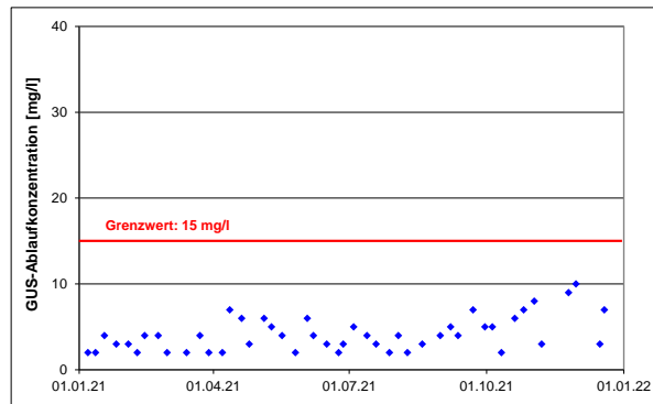
Abb. 13: Gesamte ungelöste Stoffe
