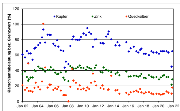
Abb. 17: Schwermetallkonzentrationen
