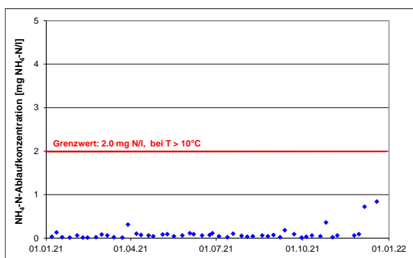
Abb. 14: Ammonium-Konzentration
