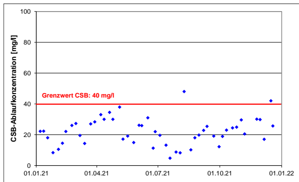
Abb. 10: CSB-Konzentration
