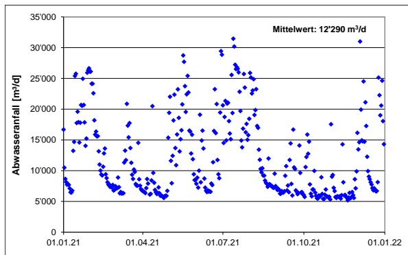
Abb. 6: Abwasseranfall
